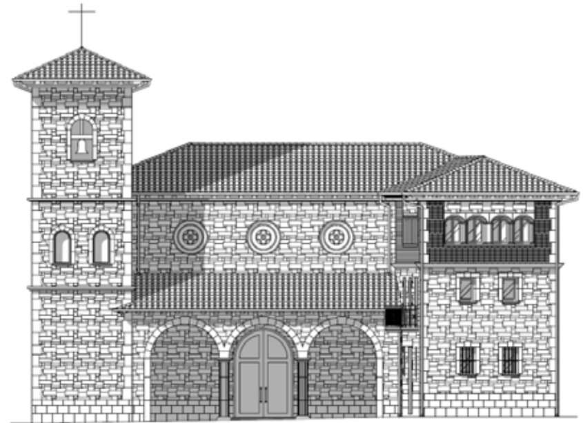
FACHADA LATERAL JARDÍN
